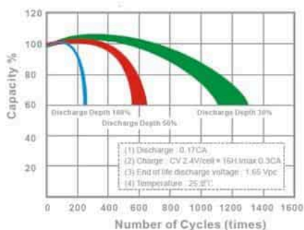
Żywotność akumulatora dla pracy cyklicznej
