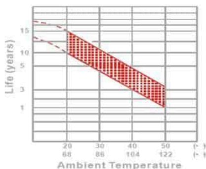
Żywotność akumulatora dla pracy cyklicznej
