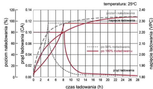
CHARAKTERYSTYKA ŁADOWANIA
