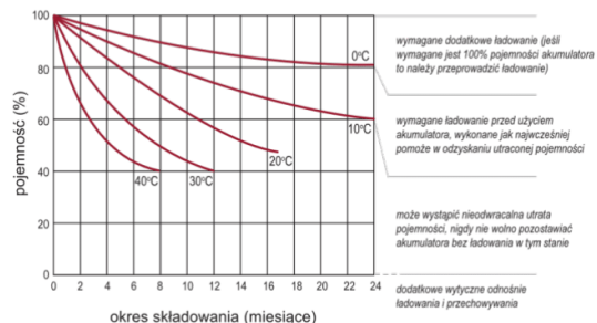
CHARAKTERYSTYKA SKŁADOWANIA
