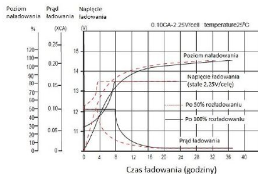
Charakterystyka ładowania - praca buforowa
