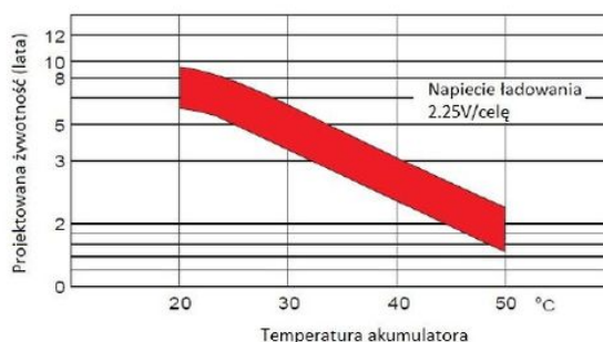
Projektowana żywotność dla pracy buforowej
